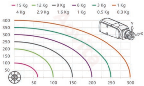
■ 负载图表
