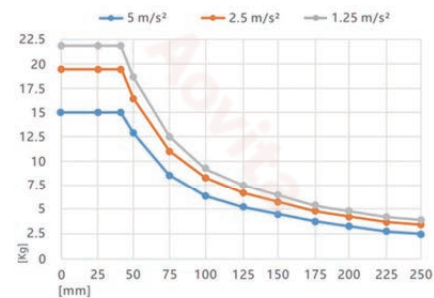
图示为最大搬运种类与加速度和力臂直接关系
