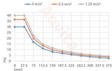
图示为最大搬运种类与加速度和力臂直接关系
