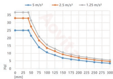
图示为最大搬运种类与加速度和力臂直接关系
