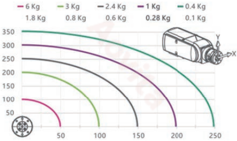
负载图表
