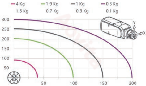
负载图表
